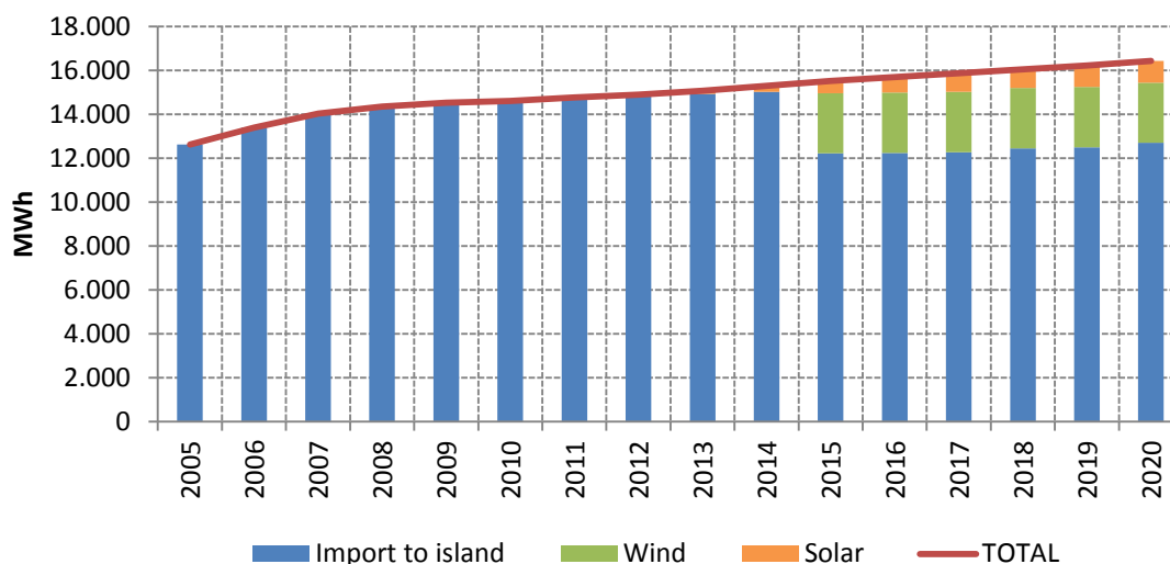
Διάγραμμα 3.35. ΝΣΔΑΕ σενάριο – Προβολή δευτερογενούς μετατροπής ενέργειας έως το 2020
