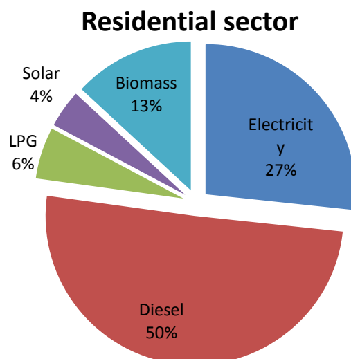
Διάγραμμα 3.2. Κατανομή της τελικής ζήτησης ενέργειας του οικιακού τομέα στους ενεργειακούς φορείς
